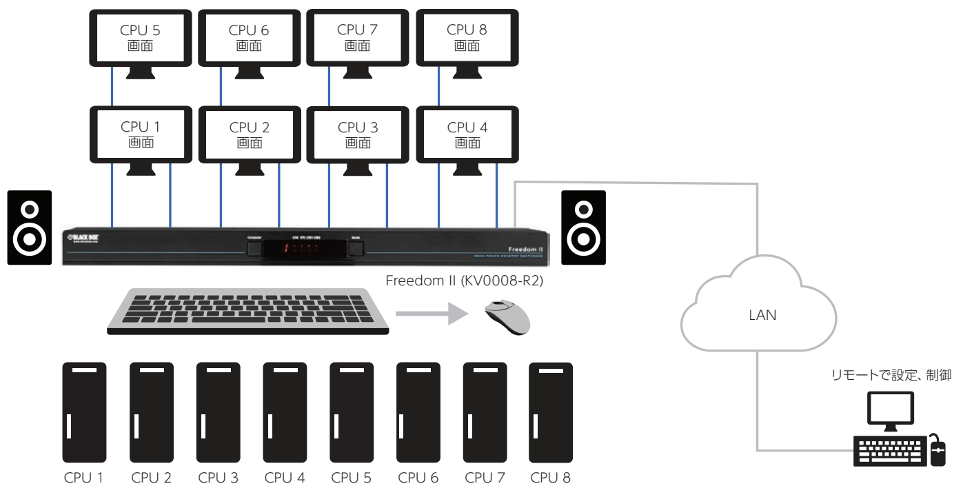
8ポート構成の Freedom II
