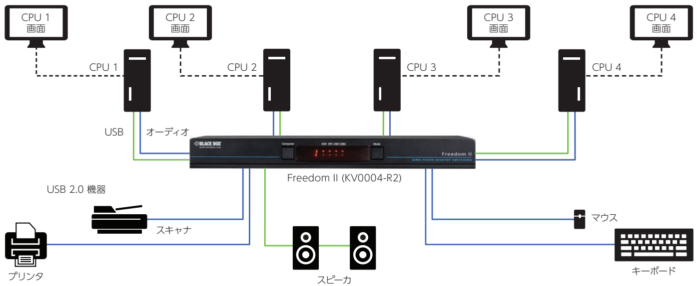
4ポート構成の Freedom II (USB 2.0 機器を含む)
