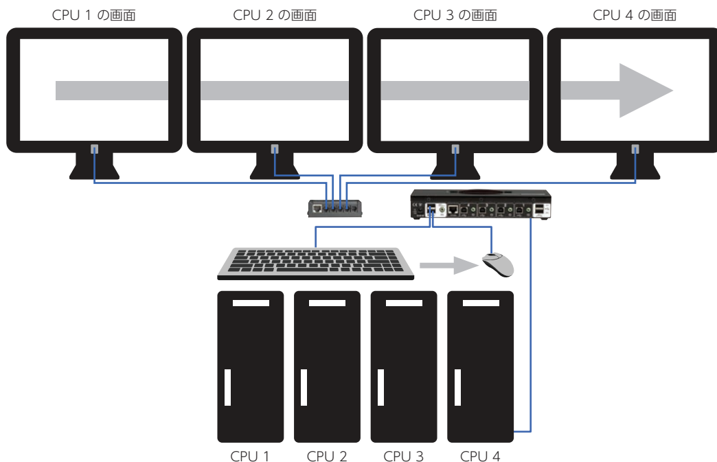
4 ポートの Freedom II スイッチと LED モニタ識別キットを使用した Glide & Switch 構成
